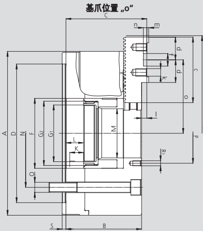
卡爪位置: 打开位置用于外夹
