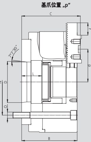
卡爪位置: 打开位置用于外夹
